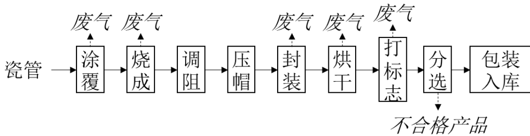
图2-2 项目 RI80 型电子元器件生产工艺流程及产污环节
