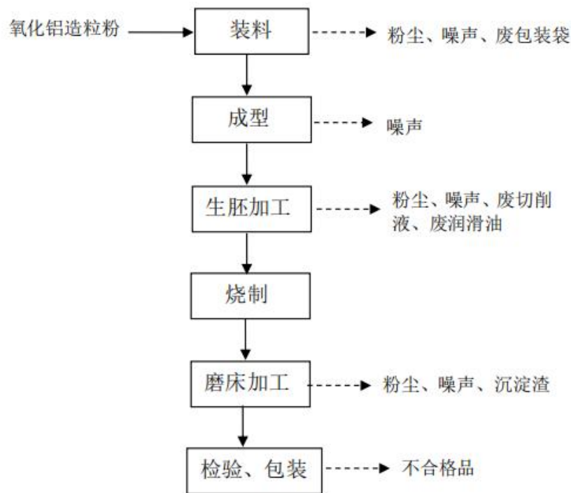
图2-2 运营期工艺流程图及产物环节图
