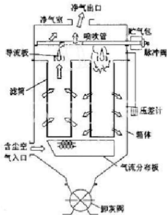
图 4-1 二级高效滤芯除尘器工作原理图
