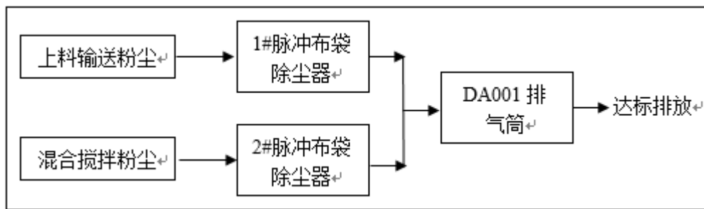
图 4-1 运营期有组织废气排放方案
