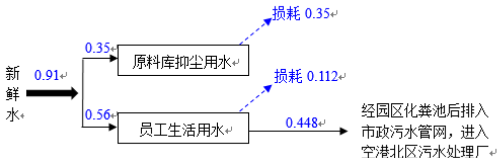
图 2-1 运营期水平衡图 单位：m 3 /d
