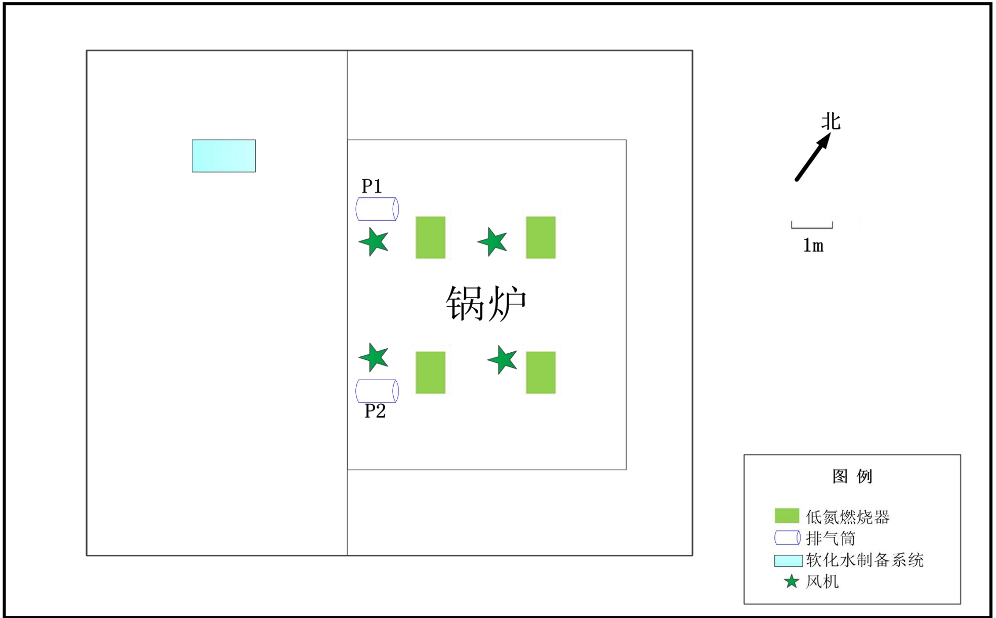
附图 4-2 项目锅炉房平面布置图
