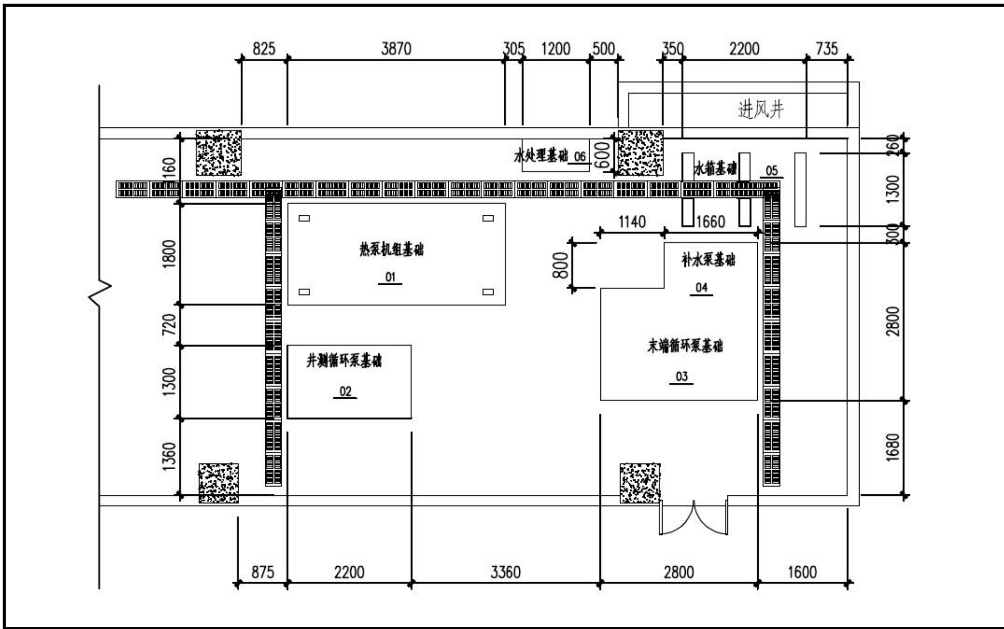
附图 4-3 项目热泵机房平面布置图
