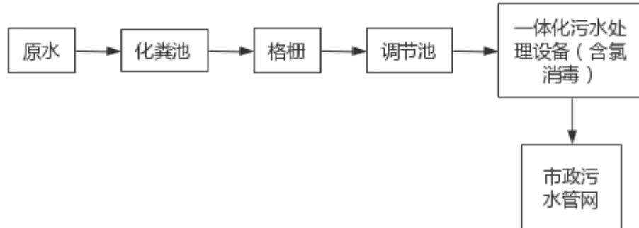
图 4-1 污水处理工艺图
