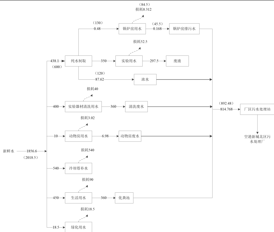
图 2-1 本项目运营期水平衡图 单位： \text{m}^3/\text{d}
