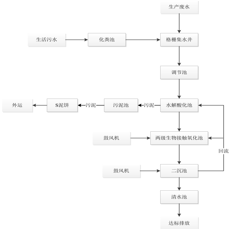
图4-1 污水处理工艺流程图
