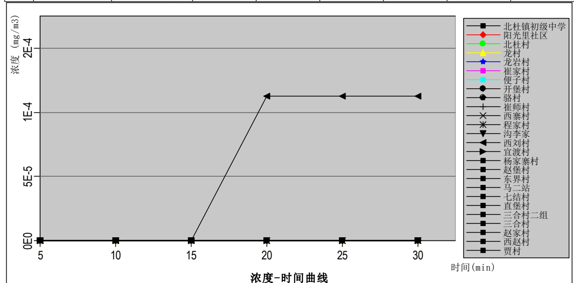
图 7.1-2 甲醇/各关心点浓度-时间曲线图
