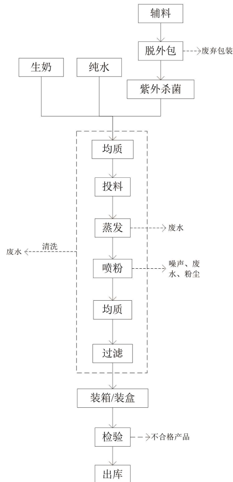
图 2-7 羊奶粉、牛奶粉、特医特膳生产线工艺流程及产污环节图
