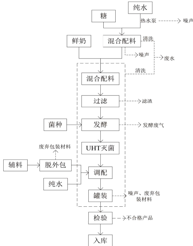
图 2-6 液态奶生产线生产工艺流程及产污环节图
