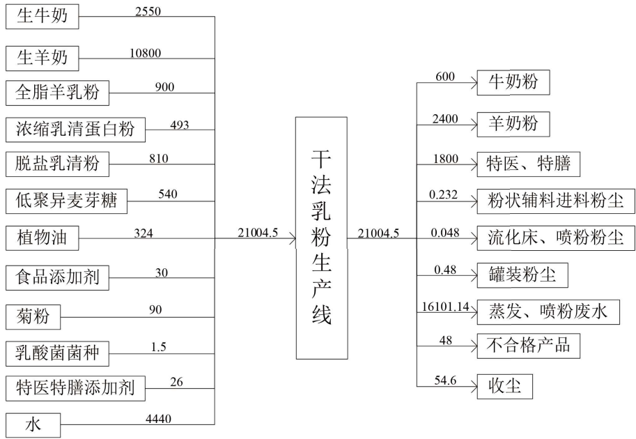
图 2-1 羊奶粉、牛奶粉、特医特膳生产线物料平衡图 (t/a)
