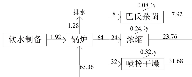
图 2-3 蒸汽平衡图 单位: m 3 /d
