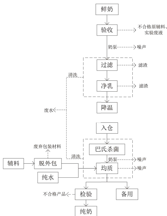
图 2-5 鲜奶前处理工艺流程及产污节点图
