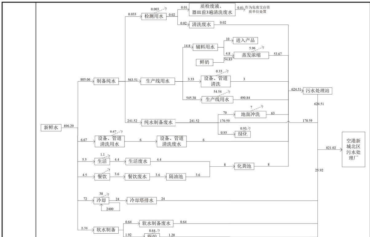
图 2-2 水平衡图单位 (m 3 /d)
