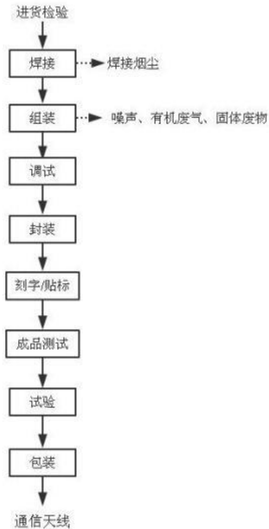
图 2-2 航天设备生产线生产工艺流程
