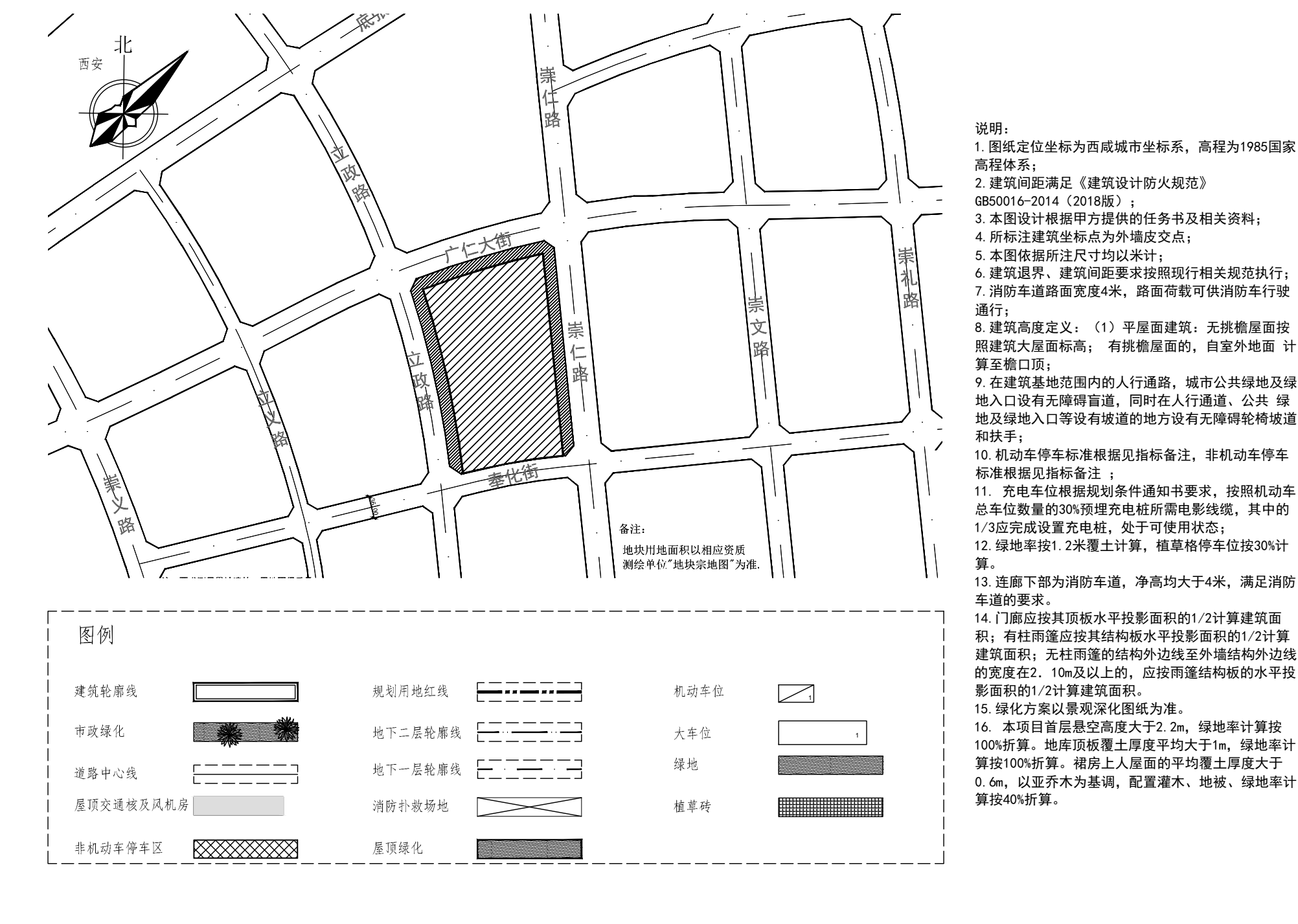
总平面图 1:500
